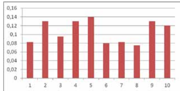
Рис. 3. Концентрация хлорофилла в вытяжках хвои
