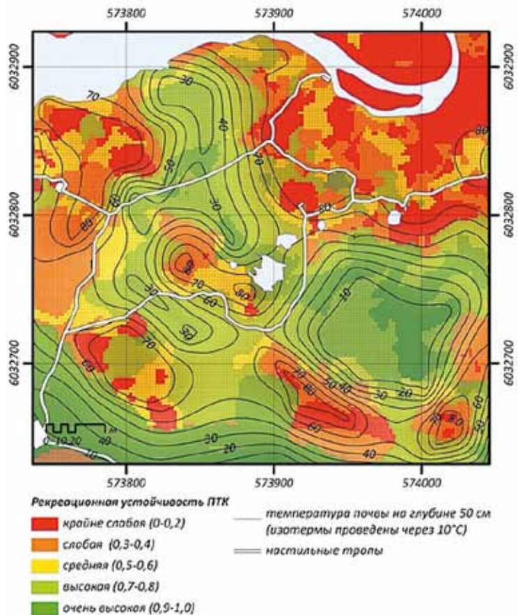
Рис. 2. Интегральная оценка рекреационной устойчивости ПТК долины р. Геизерной, сопряженная с характеристиками термальных полей
